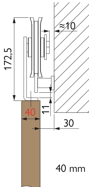
35 mm Holztür
