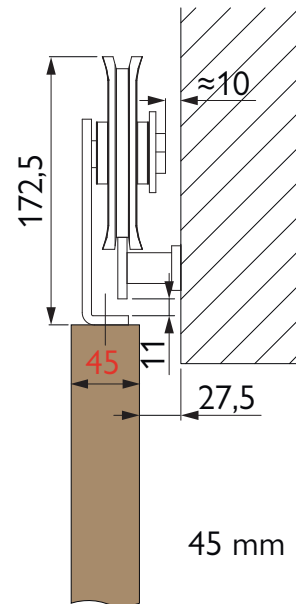
40 mm Holztür
